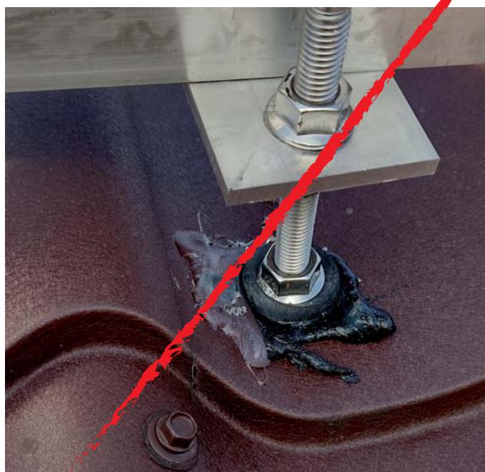
Takto NE! Kotvení FVE skrze krytinu do podkladní konstrukce má mnoho závažných rizik
